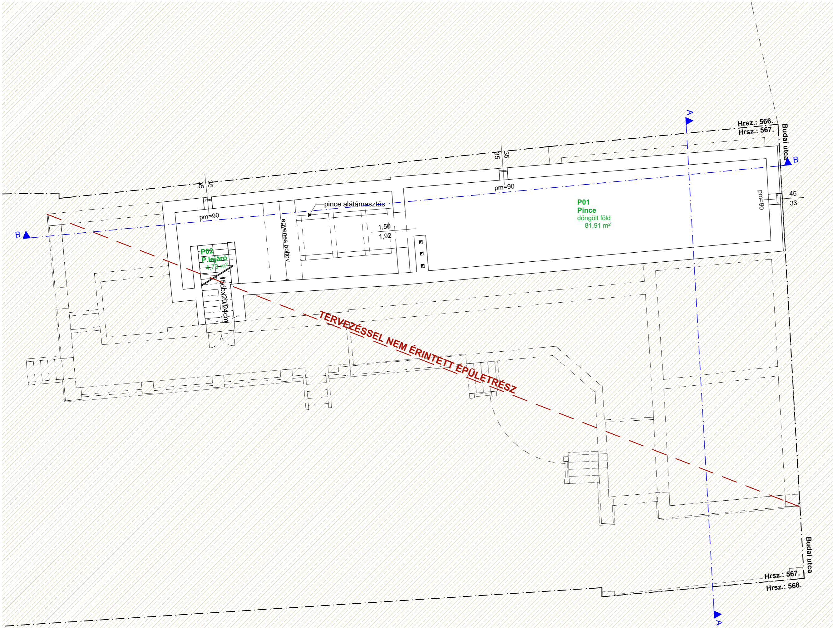
PINCESZINTI ALAPRAJZ M = 1 : 100
