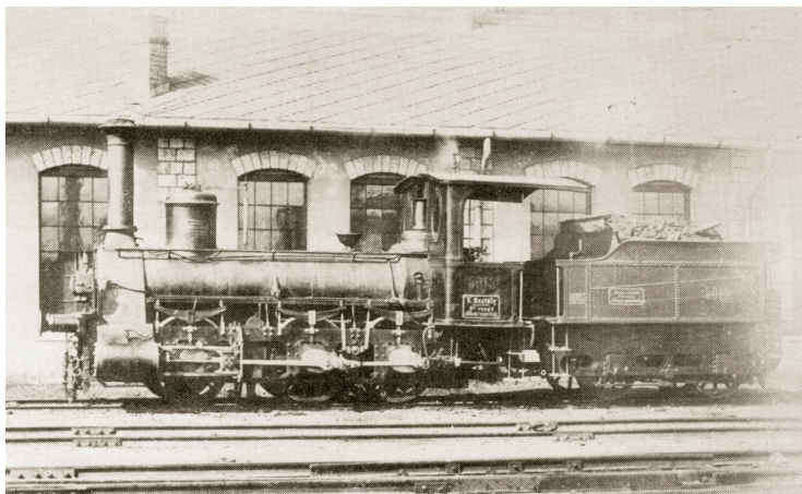
A MÁV V. osztályú szerkocsis gőzmozdony – hajdanában ilyenek járták a DDV vonalát. (forrás: Wikipedia)
