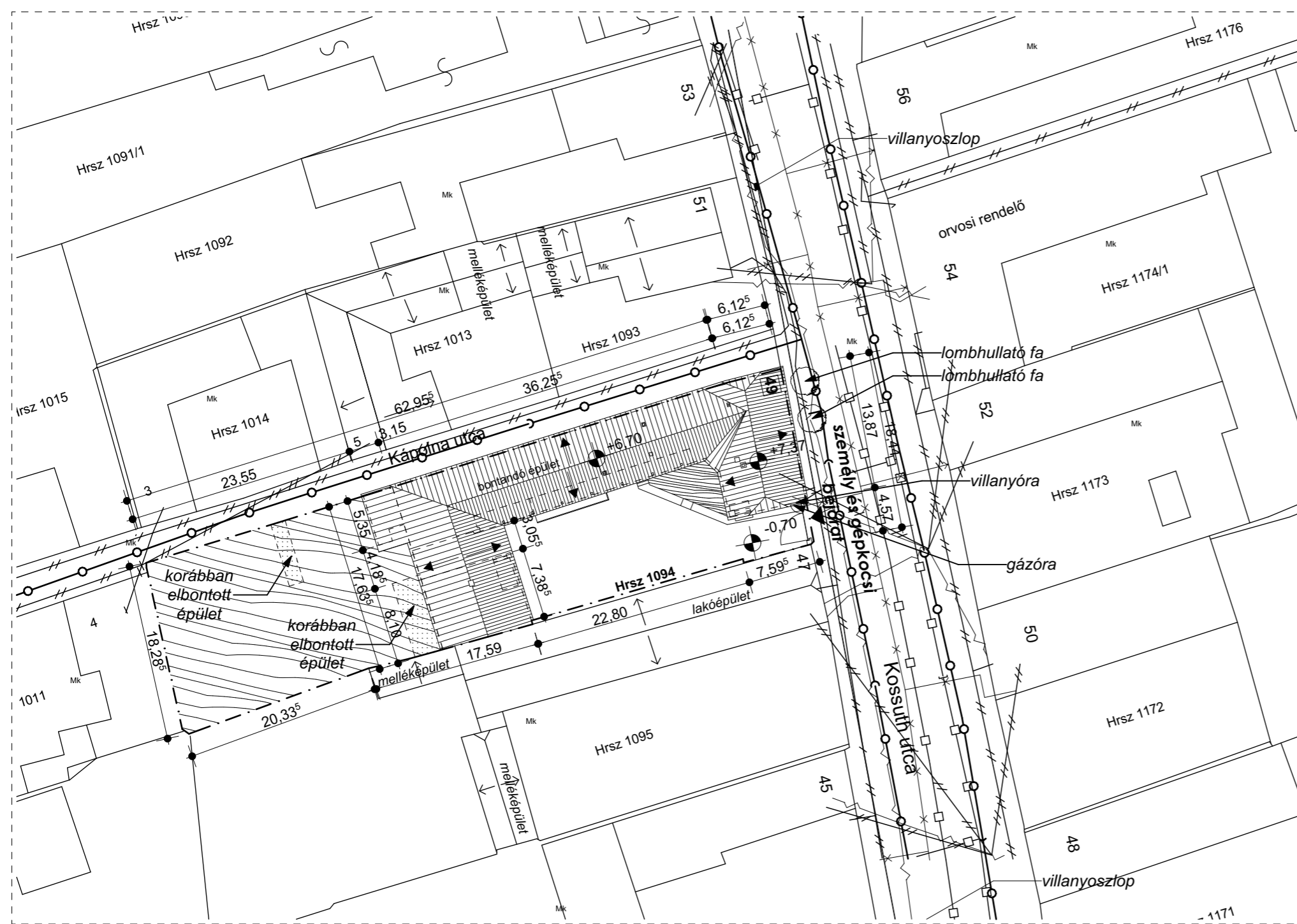
HELYSZÍNRAJZ M = 1 : 500
