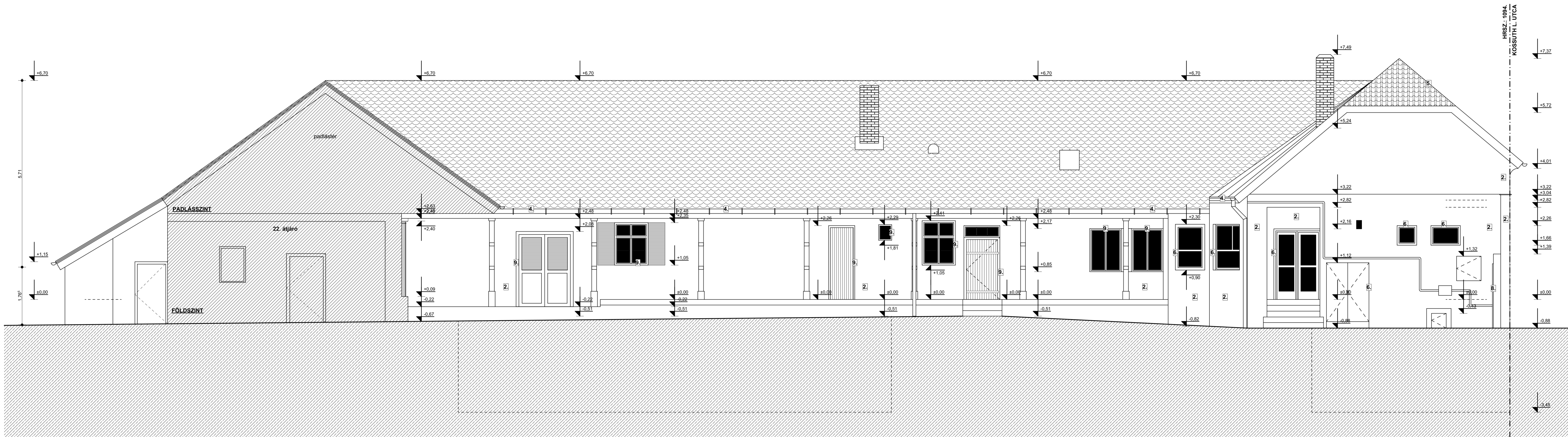
DÉLI HOMLOKZAT M = 1 : 50
