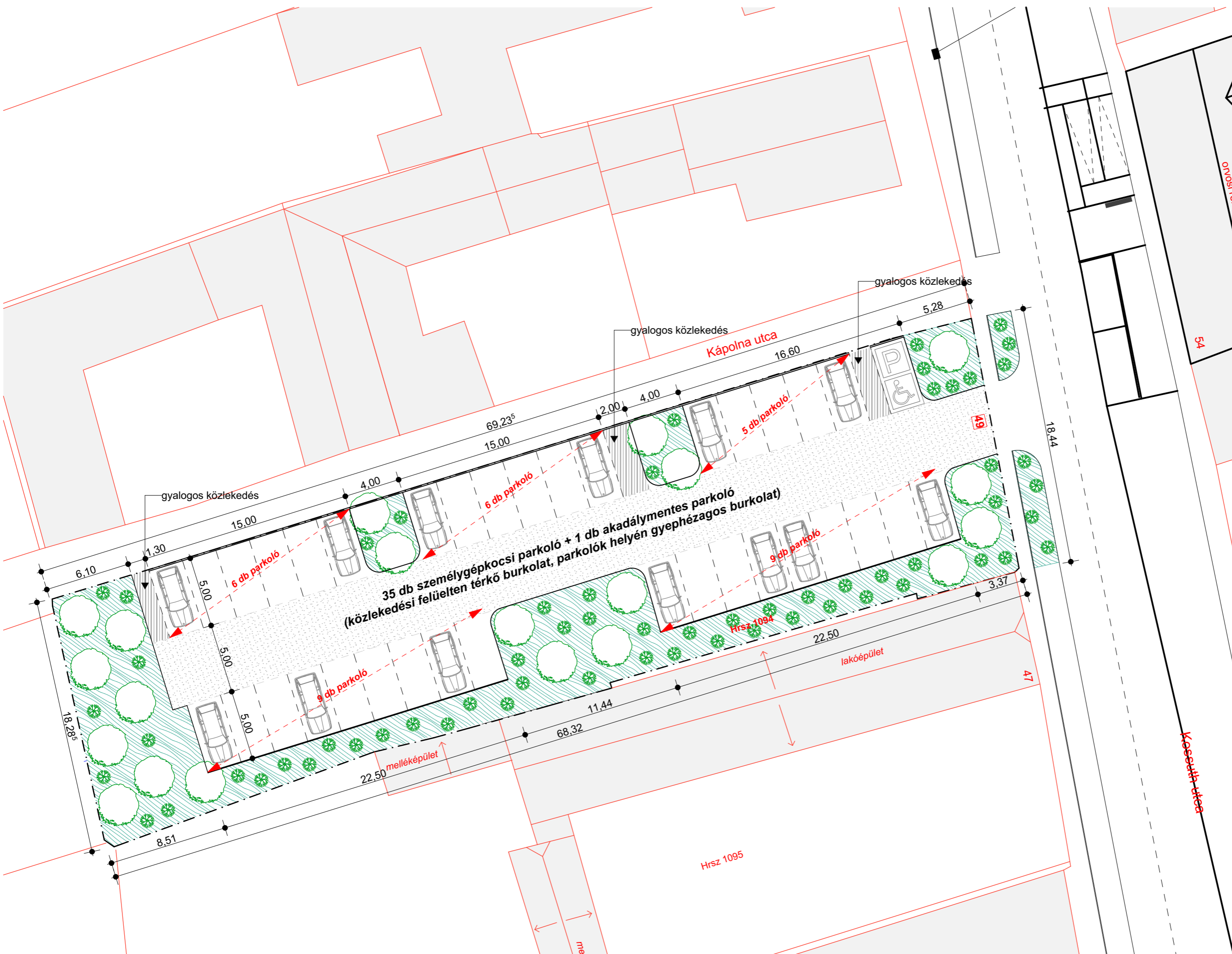
TERVEZETT PARKOLÓ KIOSZTÁS M = 1 : 250
