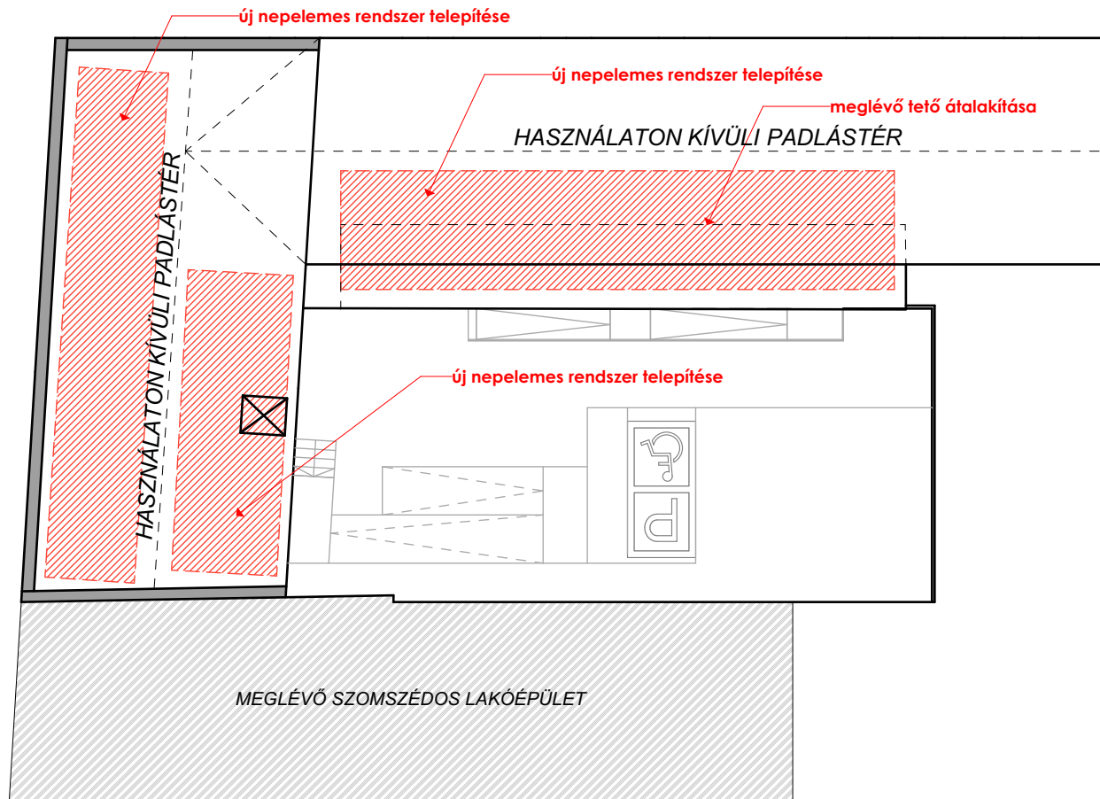
TERVEZETT PADLÁSTÉRI ALAPRAJZ M = 1 : 250
